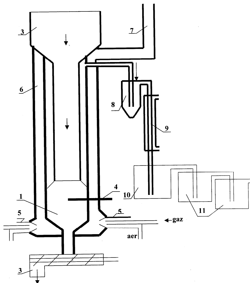
Schema instalației pentru denocivierea deșeurilor vinicole ce conțin albastru de Prusia
